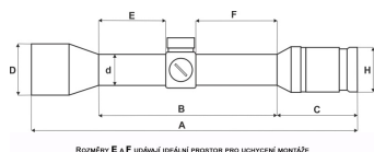
Rozměry E a F udávají ideální prostor pro uchycení montáže
